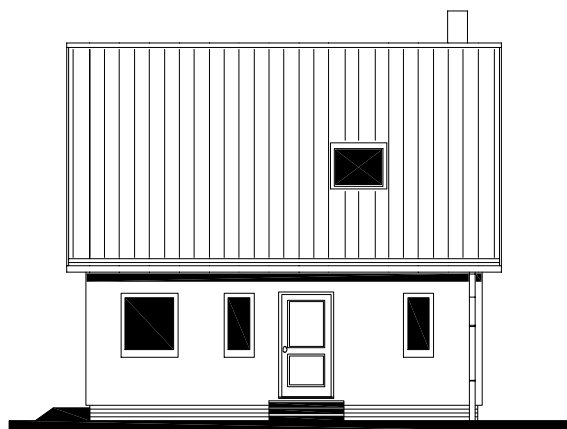
POHLED VSTUPNÍ
